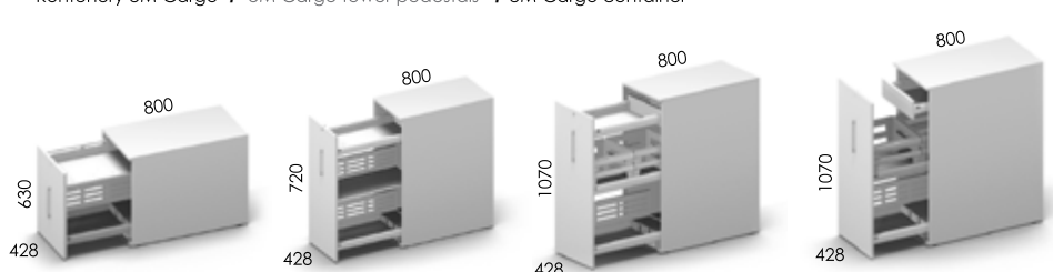
Uchwyt w kontenerze eM-Cargo Handle eM-Cargo tower pedestals Griff eM - Cargo container
