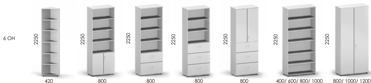
Półka metalowa z przegrodami, płytowa 25 mm, płytowa 18 mm Metal shelf, melamine shelf 25 mm melamine shelf 18 mm Metall-, Melaminfachboden 25mm, Melaminfachboden 18mm
