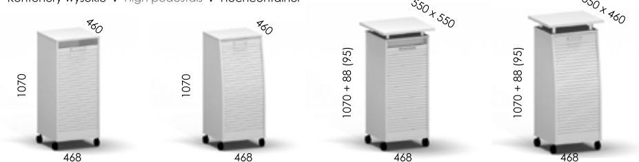
Opcja: prowadnica biała Option: white sliding guide Option: weiße Führungsschiene
