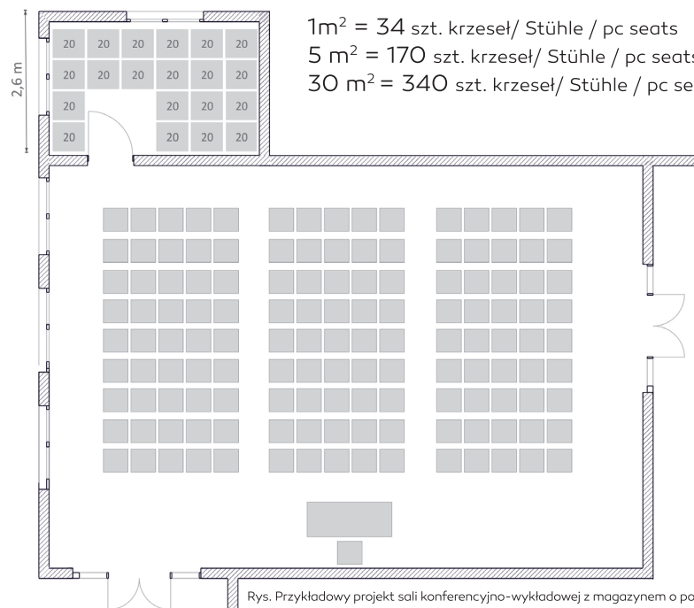
Abbildung: Beispielprojekt eines Konferenz-Vortragssaals mit einem anliegenden Lager mit einer Fläche von 12 m 2
